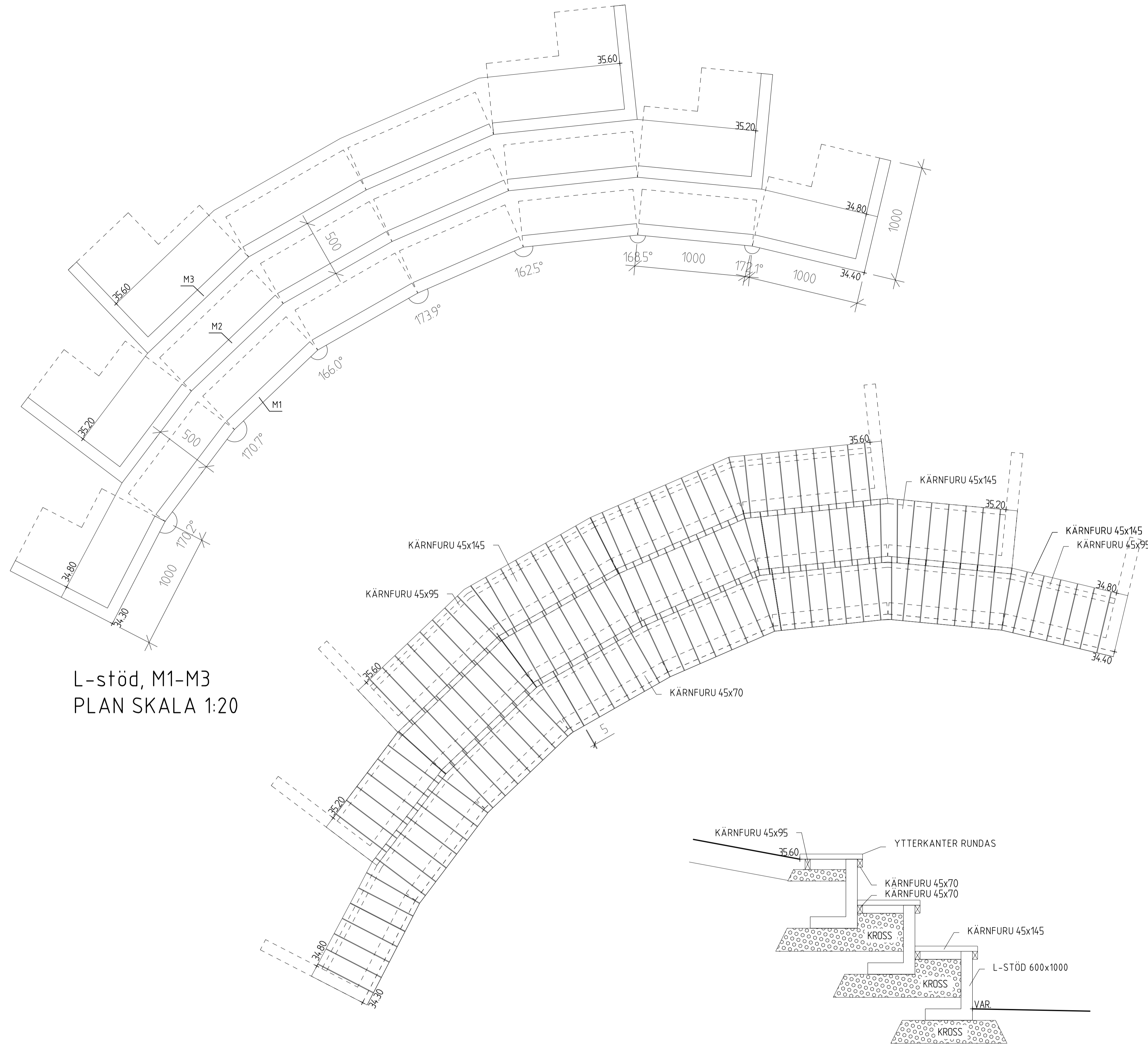
AVTÄCKNING TRÄ, L PLAN SKALA 1:20
