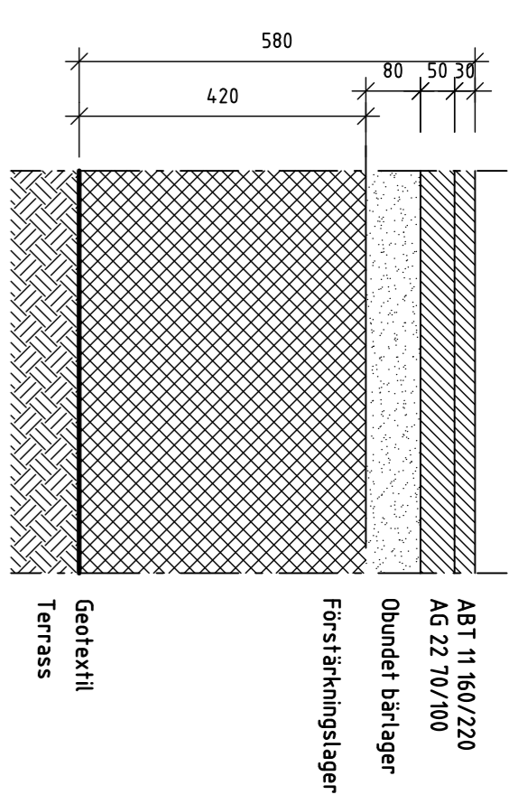
A1, SLITLAGER AV TÄT ASFALTSBETONG
