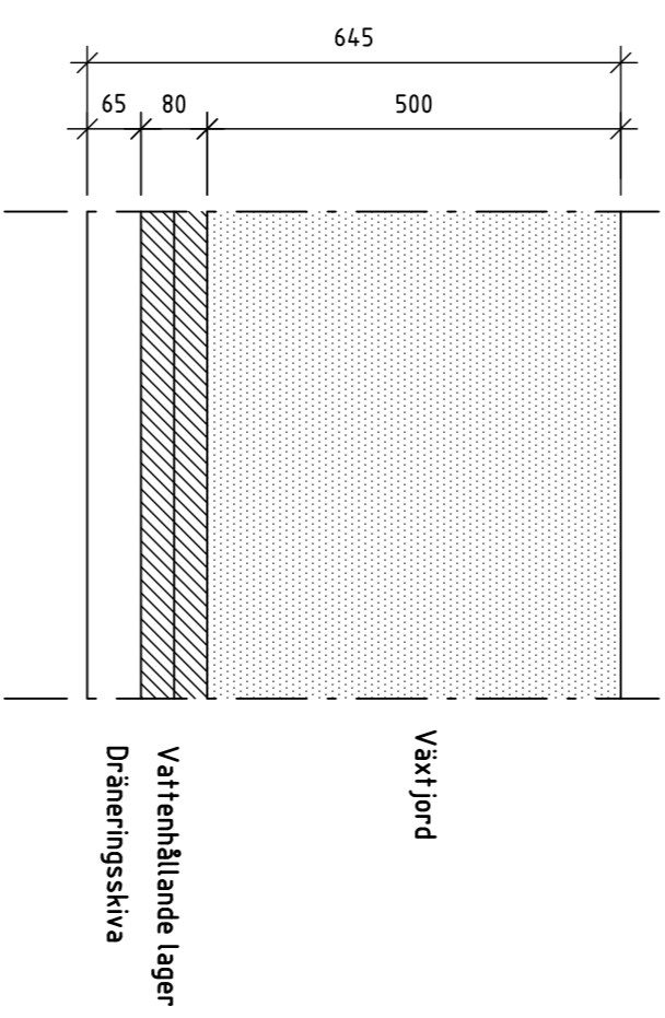
PL2, PLANTERINGSYTTA I MUR
