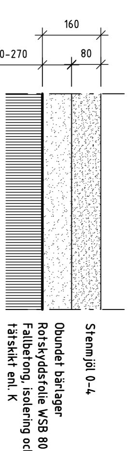
SM2, SLITLAGER AV STENMJÖL, PÅ BJÄLKLAG
