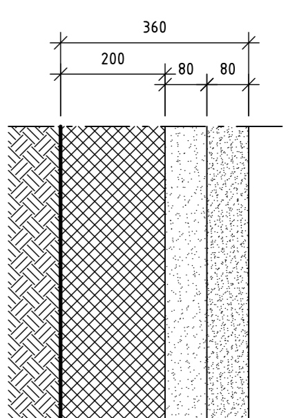
SM1, SLITLAGER AV STENMJÖL
