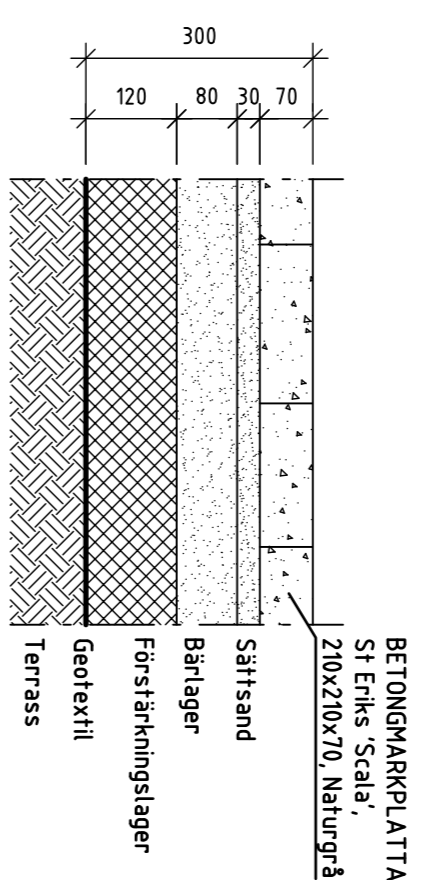
P1, BELÄGGNING AV BETONGMARKSTEN
