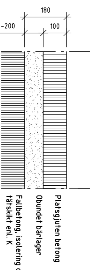
PB2, BELÄGGNING AV PLATSGJUTEN BETONG PÅ BJÄLKLAG
