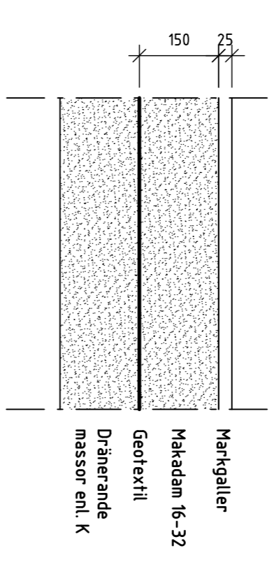
MG1, AV MARKGALLER
