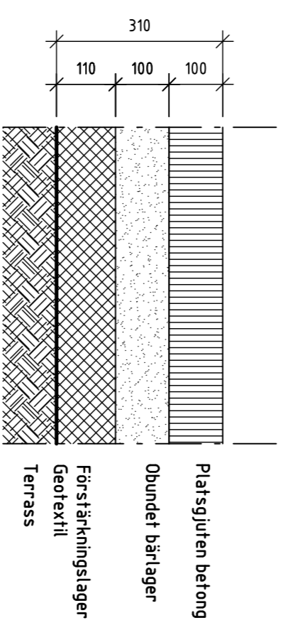
PB1, BELÄGGNING AV PLATSGJUTEN BETONG
