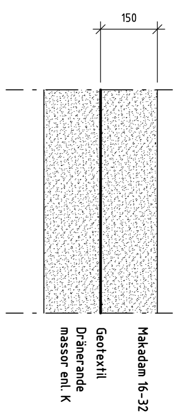
G1, SLITLAGER AV GRUS
