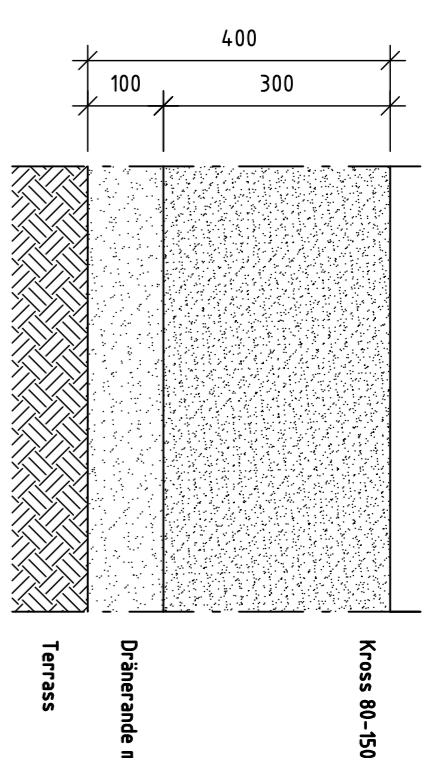
G3 BELÄGGNING AV KROSS
