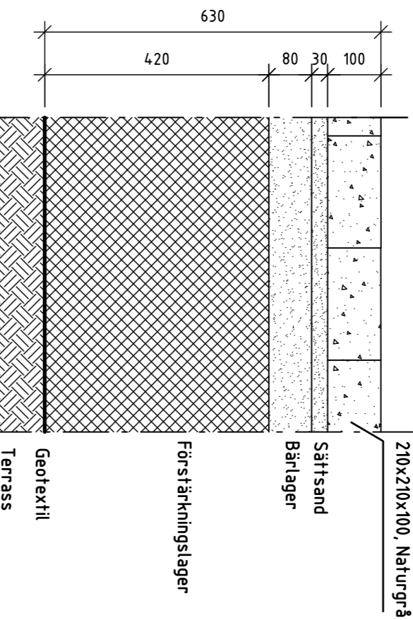
P3, BELÄGGNING AV BETONGMARKSTEN
