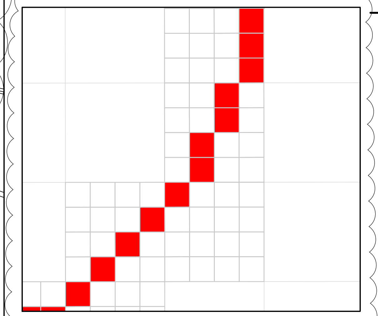
DETALJ PRINCIP MÖTE MUNKSTEN 105x105 MED MUNKSTEN 420x420 PLAN, Skala 1:10
