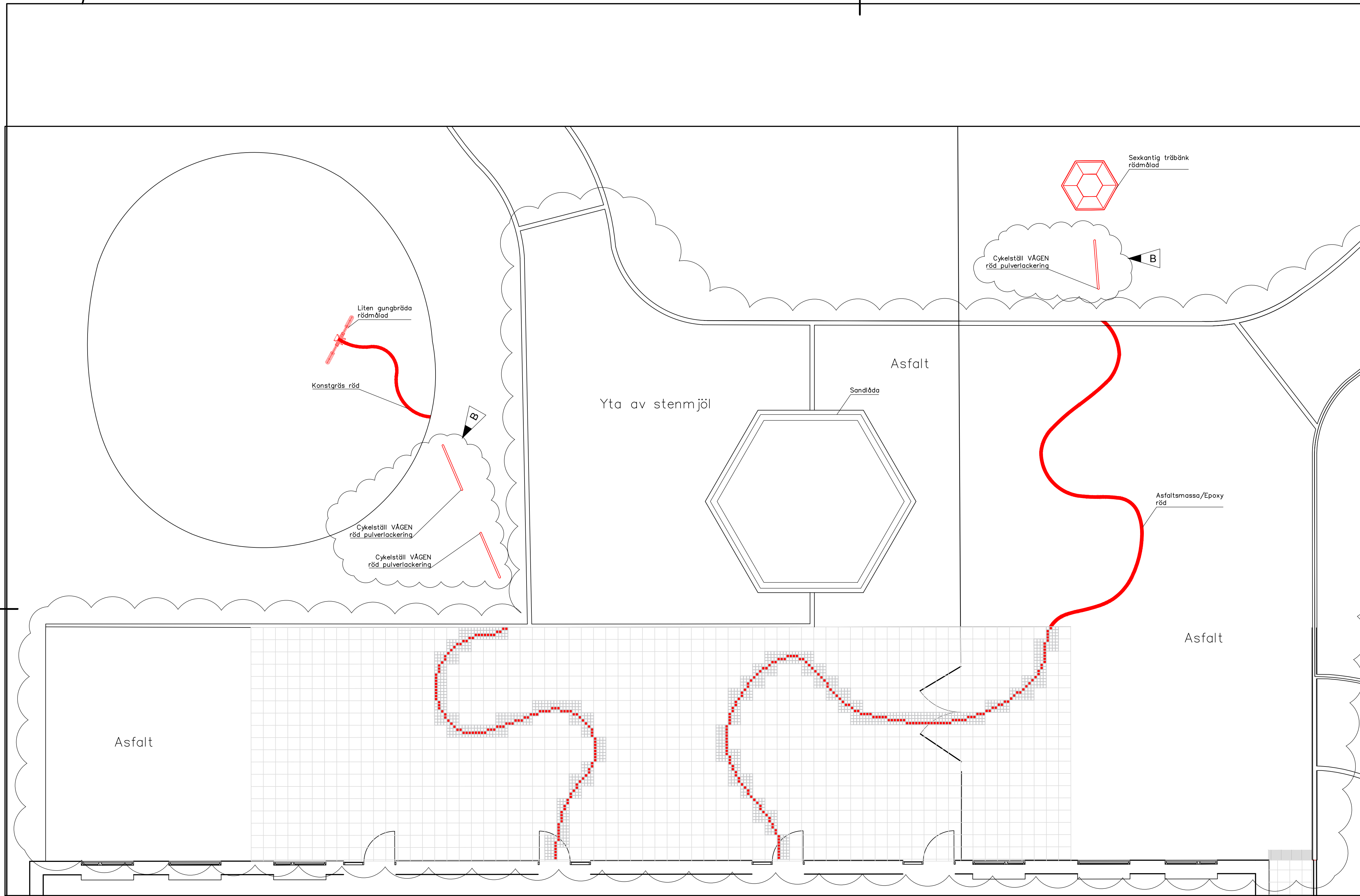
DETALJ MARKBELÄGGNING BTG1 OCH BTG2 PLAN, Skala 1:75
