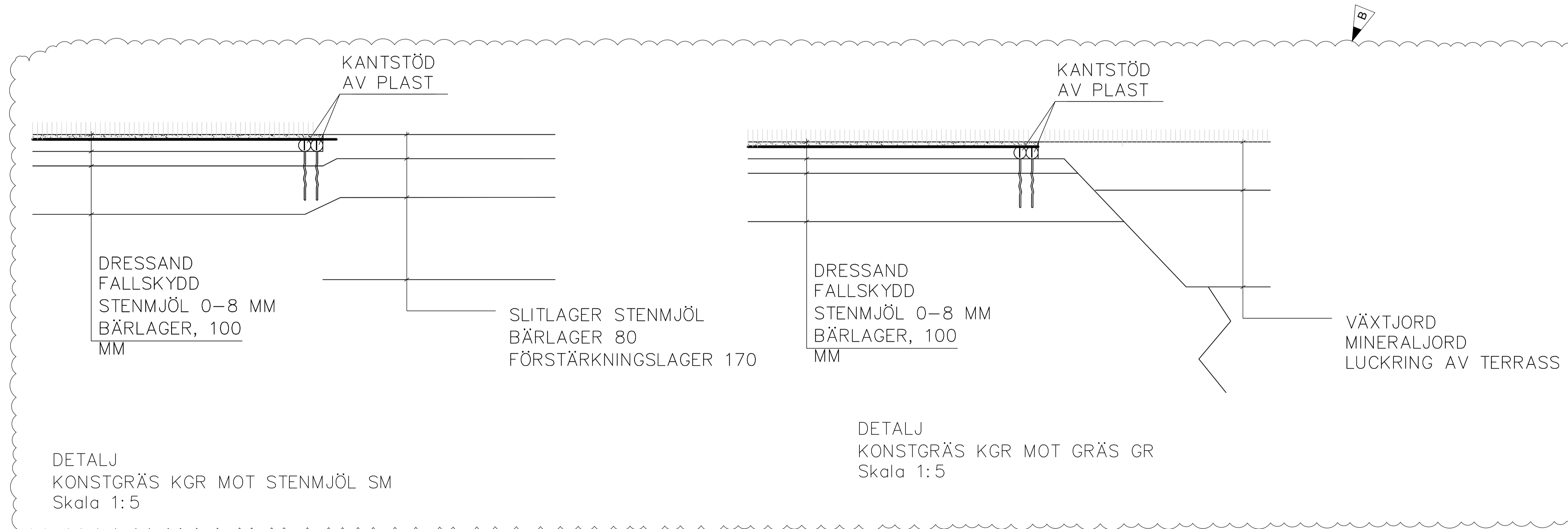
DETALJ FRIS AV STORGATSTEN F1 Skala 1:10
